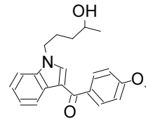
54 RCS-4 N-(4-...
