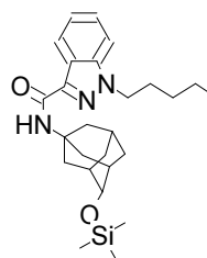
111 AKB48-M1-...
