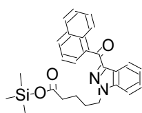
112 THJ-2201 M...
