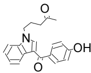
52 RCS-4 M11 ...
