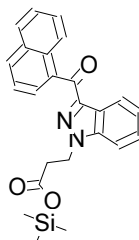
113 THJ-2201 M...
