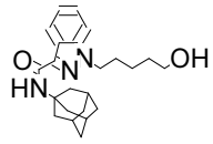
13 AKB48 N-(5-...
