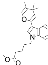
120 XLR11 (-F, ...
