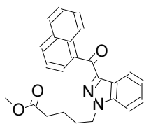
115 THJ-2201-M...
