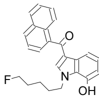
16 AM2201 7-hy...
