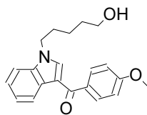
55 RCS-4 N-(5-...
