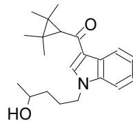
56 UR-144 N-(4-...
