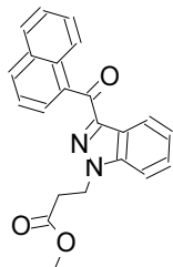
109 THJ2201-M...
