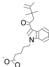
119 XLR11 M28 ...
