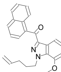
117 THJ-2201-M...
