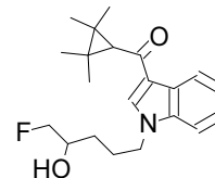
57 XLR11 N-(4-...
