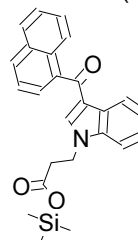
114 AM-2201 (-...
