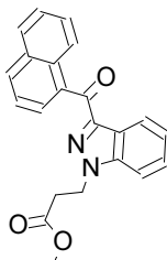
116 THJ-2201-M...
