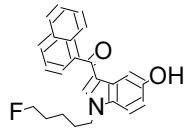
14 AM2201 5-hy...
