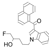
17 AM2201 N-(4...
