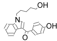
51 RCS-4 M10 ...
